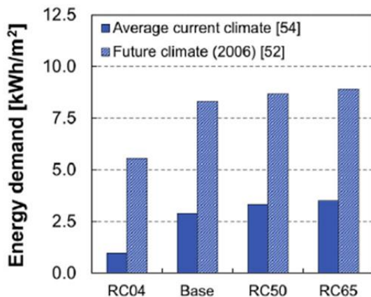
Figuur 4 Elektriciteitsvraag voor koeling, vergelijking van het huidige klimaat en toekomstige klimaat voor vier gebouwvarianten met toenemende gevelisolatie. (RC= Rc-waarde voor dichte gevel) [15]
