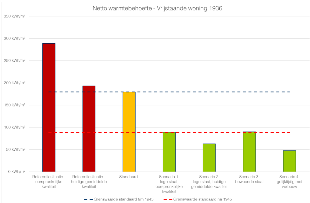
Figuur 10: Netto-warmtebehoefte per scenario vrijstaande woning – 1936
